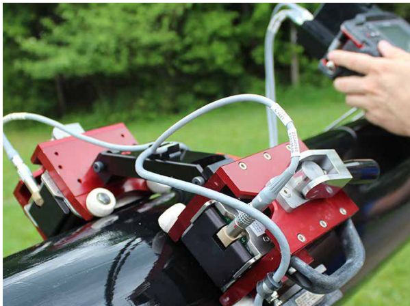
การทดสอบโดยคลื่นเสียงความถี่สูงแบบระยะทดสอบปานกลาง (Medium Range Ultrasonic Test)
